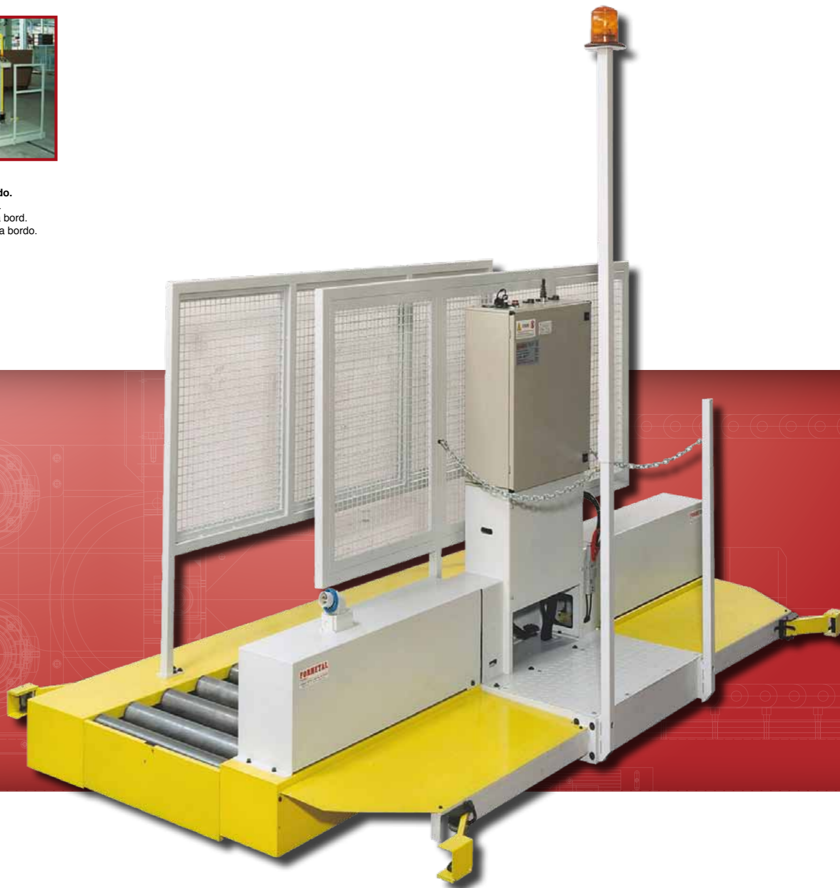
Navetta traslante con uomo a bordo. Travelling shuttle with man on board. Navette translateur avec operateur à bord. Navecilla de transporte con hombre a bordo.
